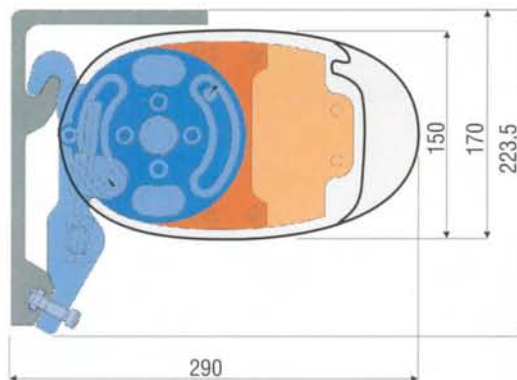
Markise mit Kombikonsole Decke/Wand
